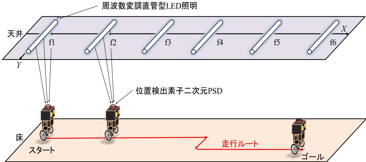
周波数変調LED照明によってガイドされる無人搬送車の走行イメージ
